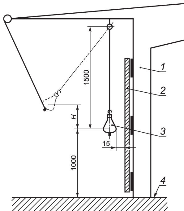
Рисунок ДА.1 — Маятник для нежесткого удара
