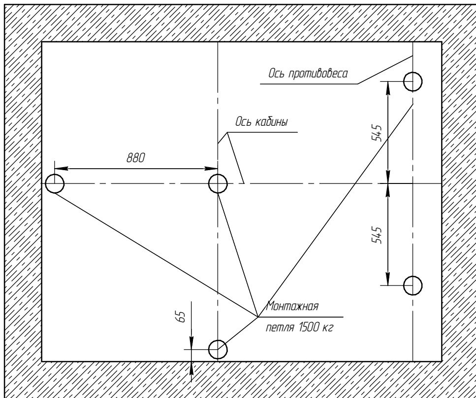
В-В (1:20)
