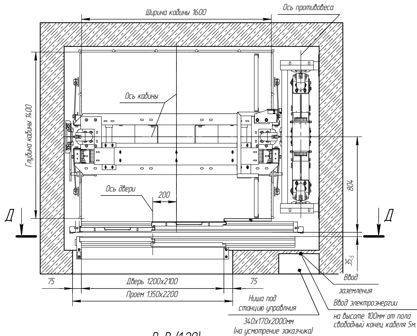
В-В (1:20)
