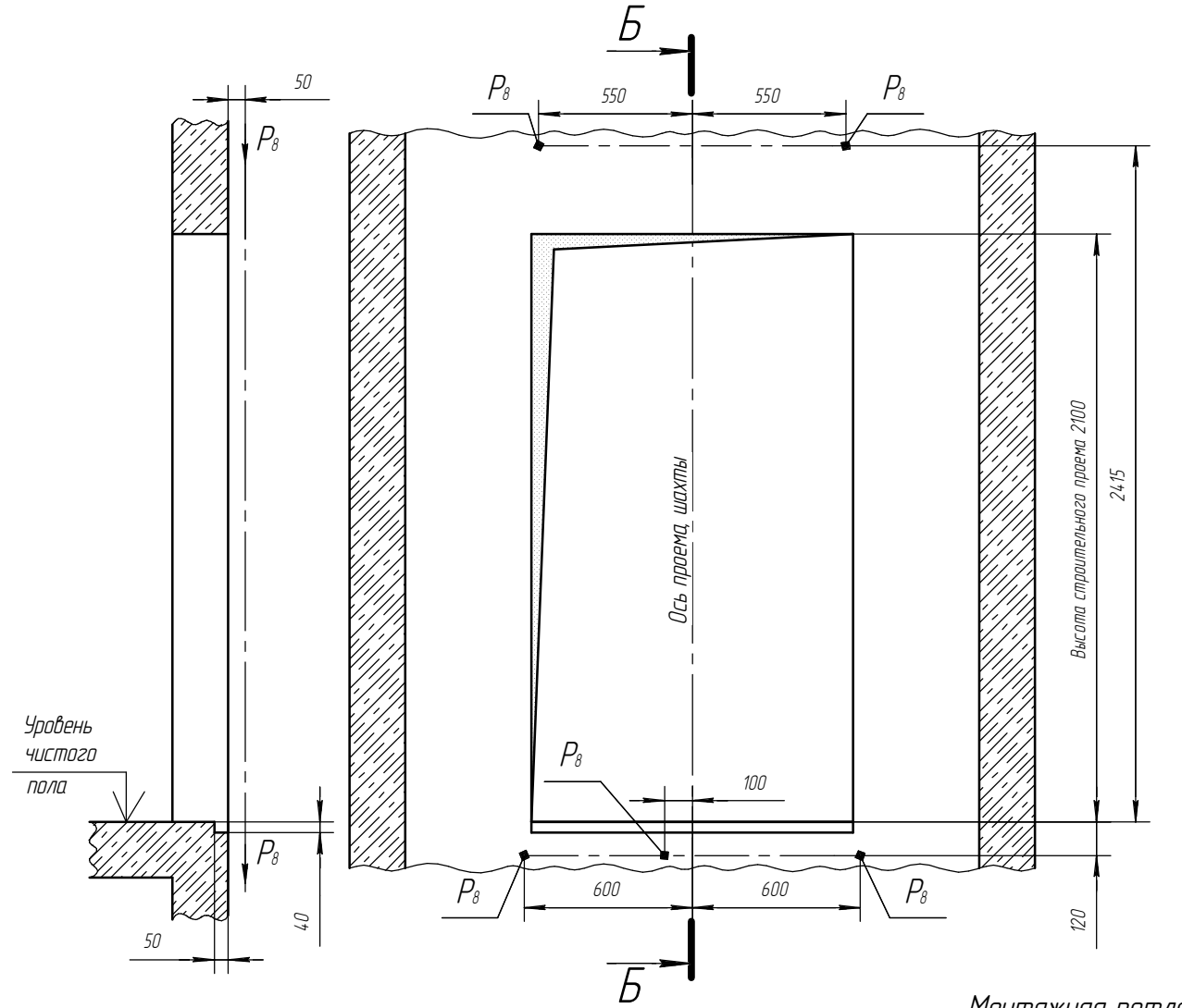
Монтажная петля 2 места
