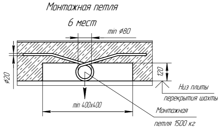
Е(1:10)(1)
